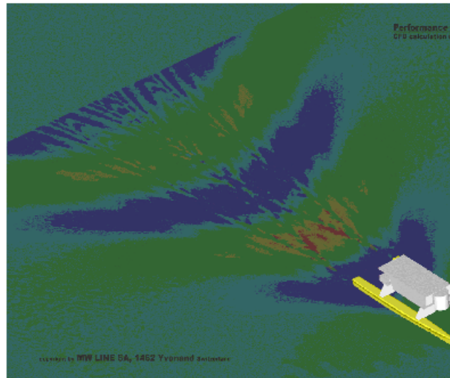
Champ du relief des vagues autour du C100, un projet de ferry solaire pour 100 personnes, développé par la société MW-Line
