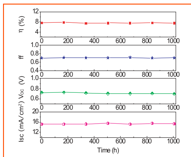
Figure 4 - Effet du vieillissement à 80-85 °C pendant une période de 1000 h sur les paramètres photovoltaïques de cellules à colorant [5].
