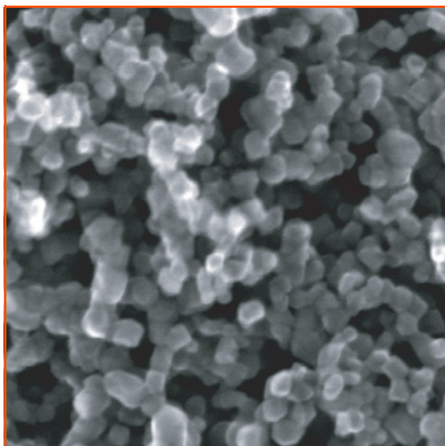
Figure 2 - Image d'une couche mésoscopique du dioxyde de titane déposée sur un verre conducteur. Chaque grain constitue un nanocristal d'une taille d'environ 20 nm.
